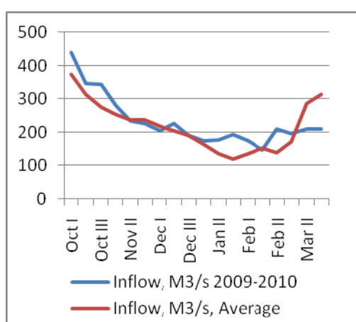
Приток в Нурек-ом водохранилище, в куб. м. / сек
