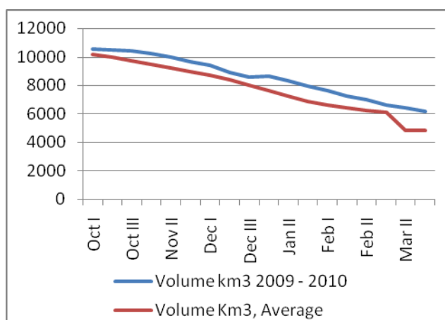
Объем воды в Нурек-ом водохранилище, в куб. м.
